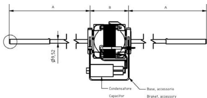
Motori 4 POLI - MULTIVELOCITÀ / 4 POLES - MULTISPEED MOTORS
